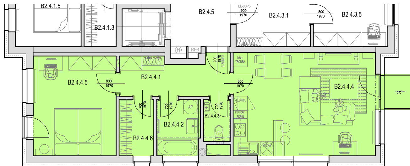
schéma podlaží
