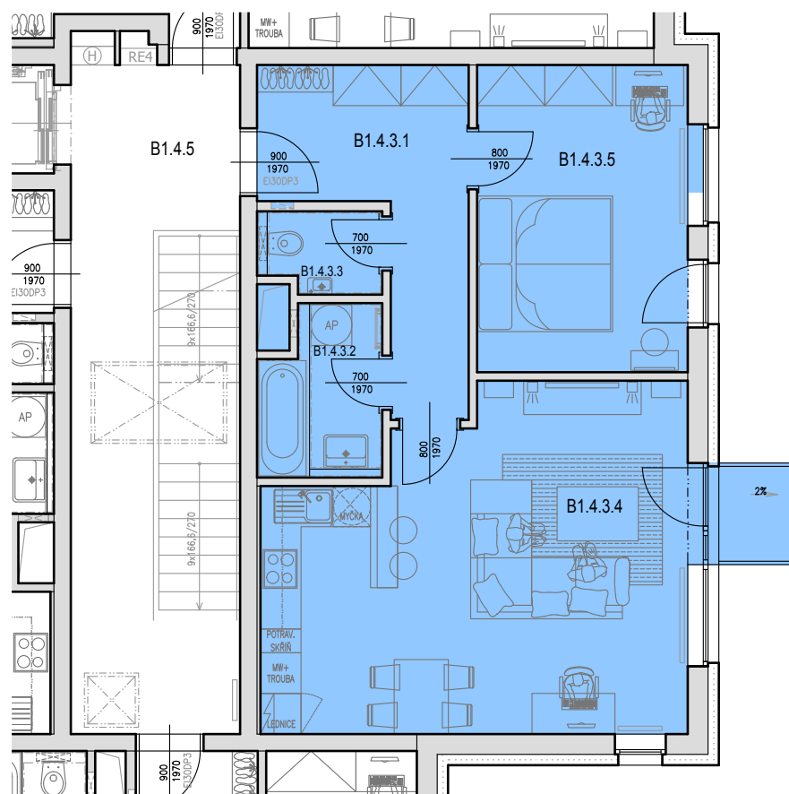
schéma podlaží
