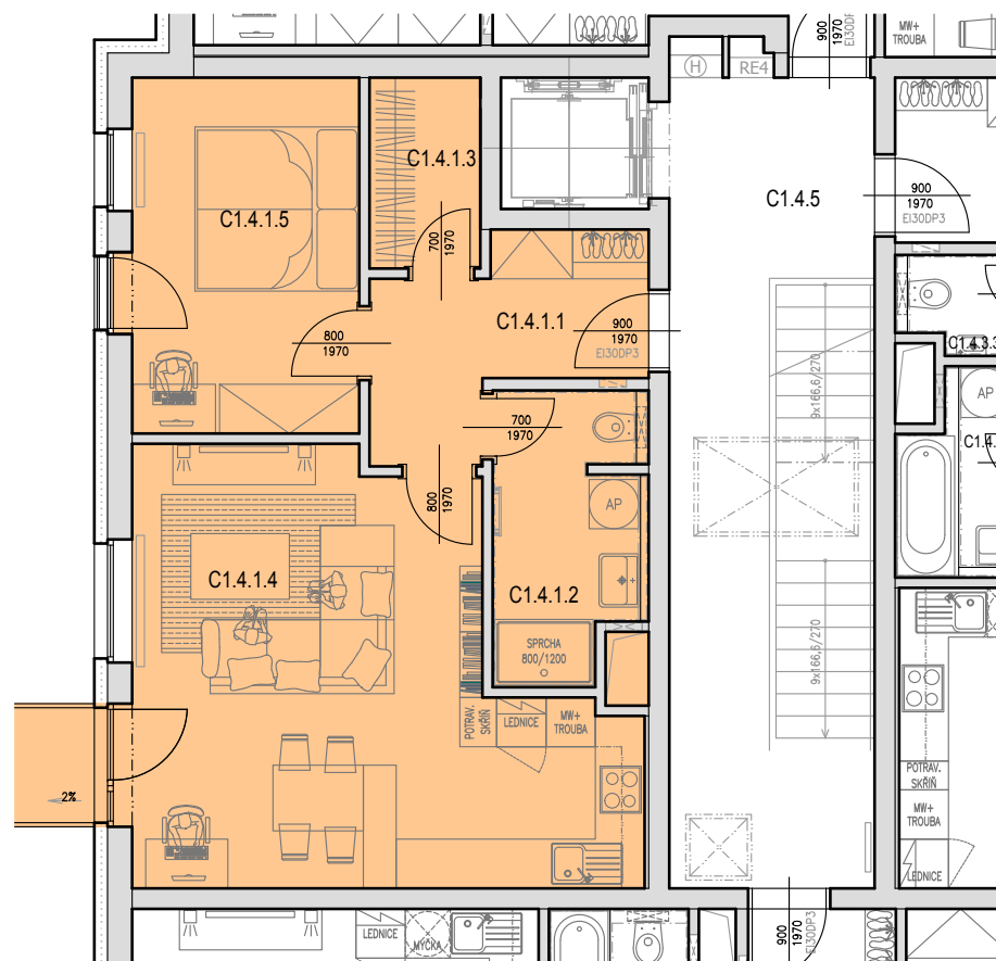
schéma podlaží
